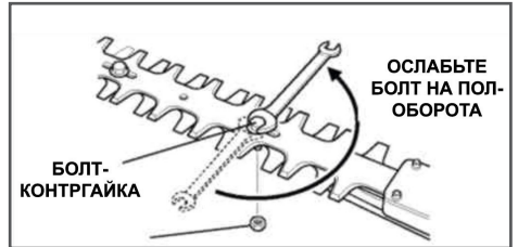
Рис. 12 Затачивание ножей (А): 6 мм радиус (В): 100° (прибл.) (С): 45°
